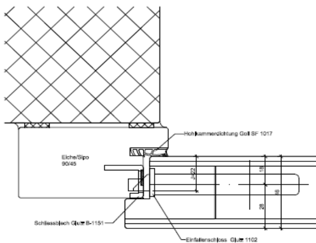
A-A Detail Schloss
